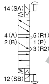
ABR connection
